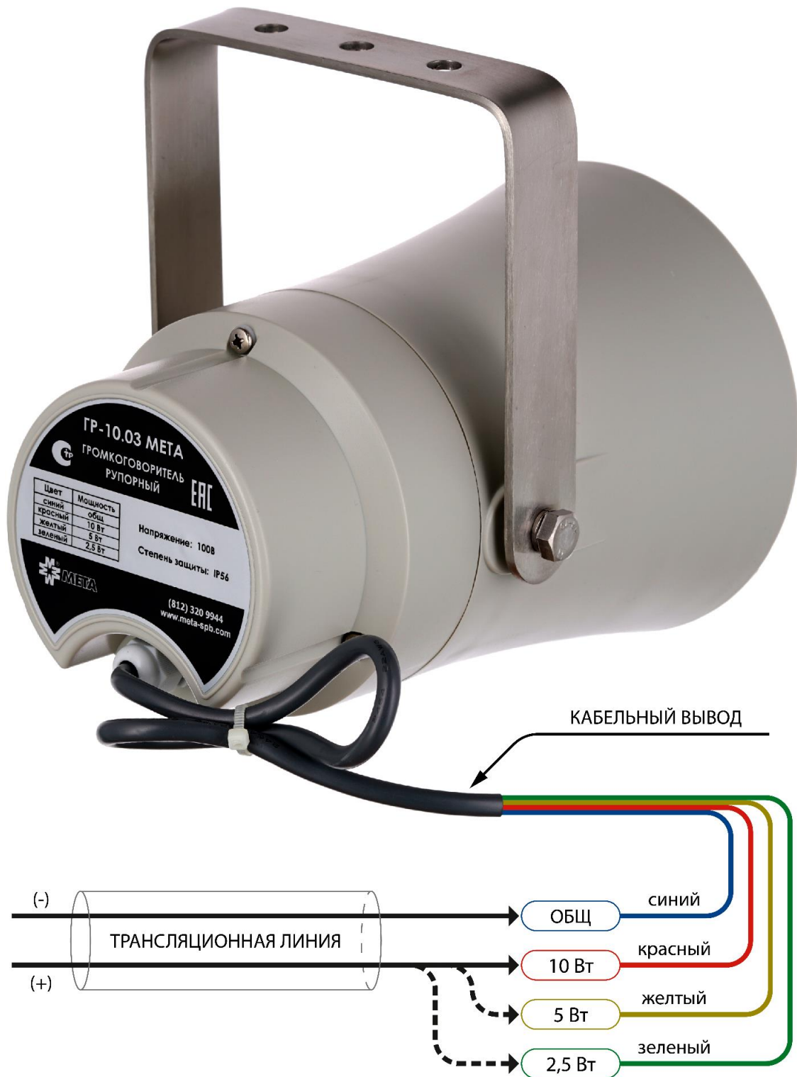
Рис.3 Схема подключения ГР к трансляционной линии.
