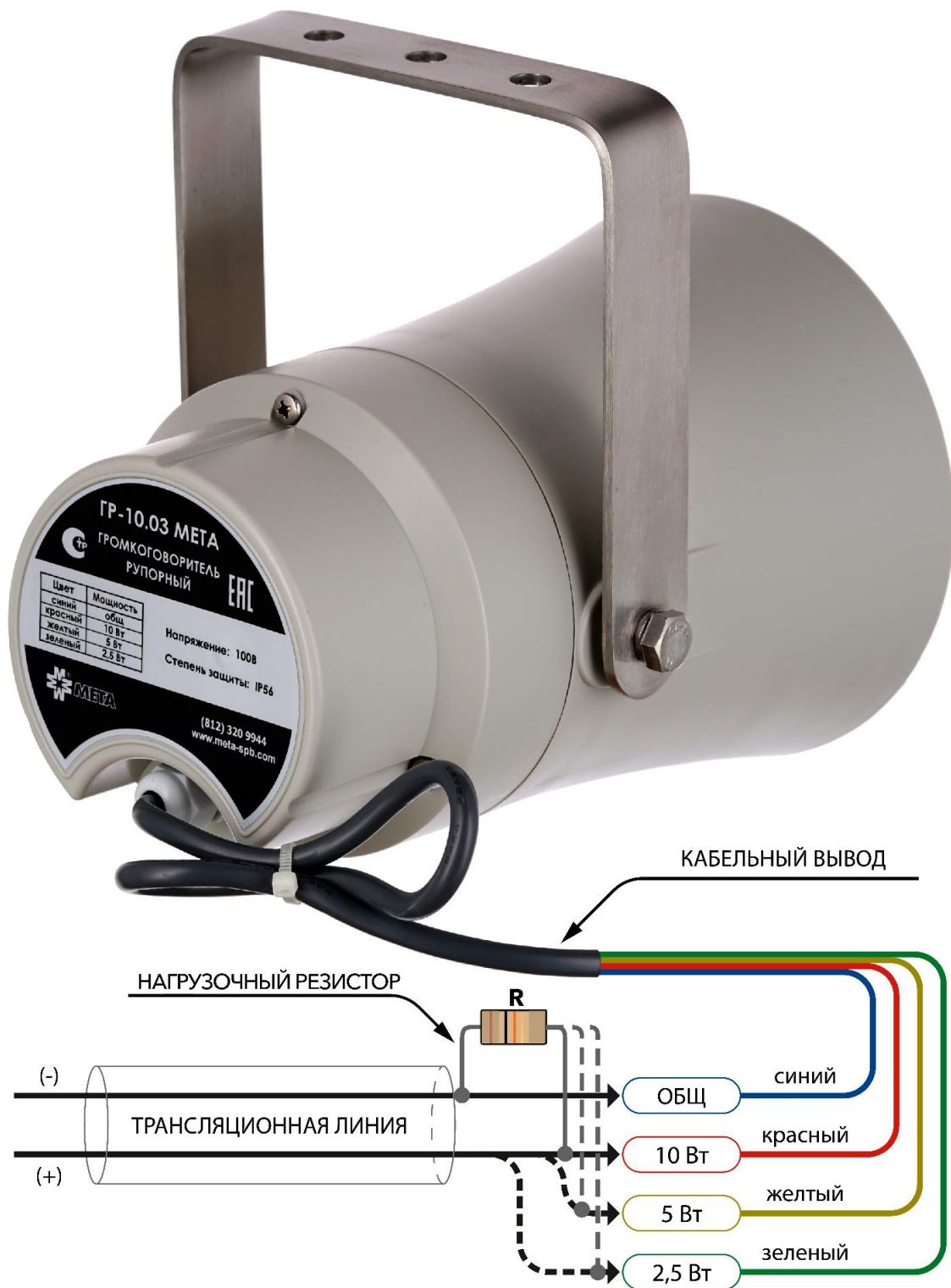
Рис.4 Схема подключения нагрузочного резистора к ГР-10.03 МЕТА исп.3.
