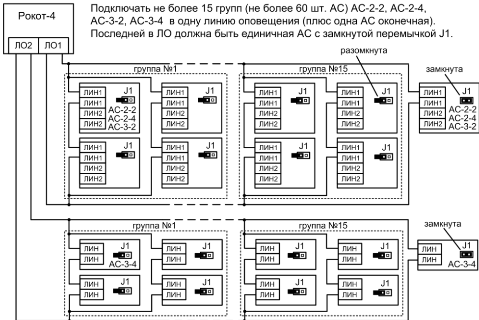
Рис.А5 Схема подключения акустических систем «АС-2-2», «АС-2-4», «АС-3-2» и «АС-3-4» (параллельное соединение групп АС)
