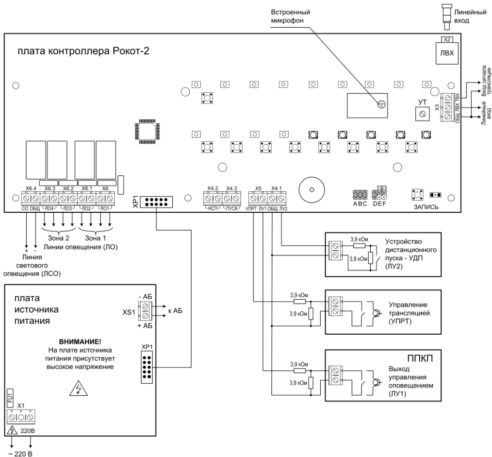
Рис.А1 Плата контроллера (вид со снятой панелью индикации и управления), плата источника питания и схемы внешних подключений прибора «Рокот-2»
