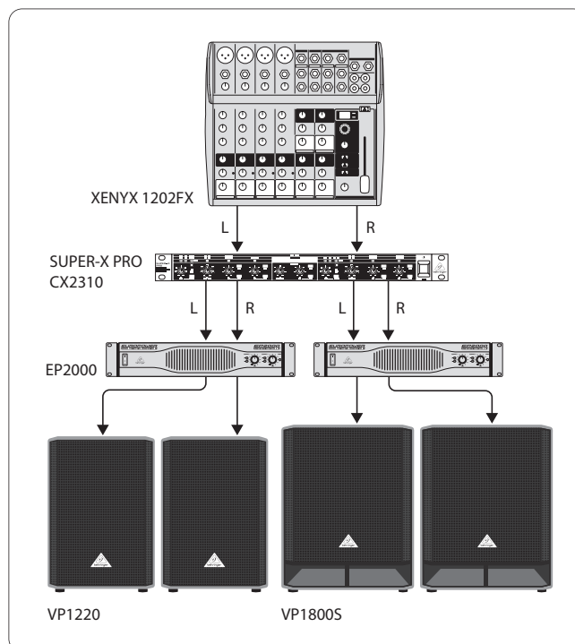
Фиг. 5.3: Двухканальный стереофонический режим с сабвуферами
