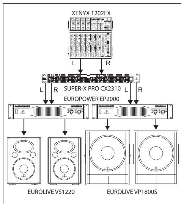
Фиг. 5.3. Двухканальный стереофонический режим с сабвуферами
