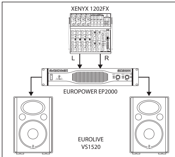
Фиг. 5.1. Стерефонический режим с полным частотным диапазоном
