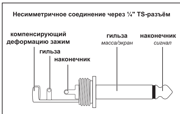
Фиг. 2.3. Разъем TS для громкоговорителей размером ¼ дюйма
