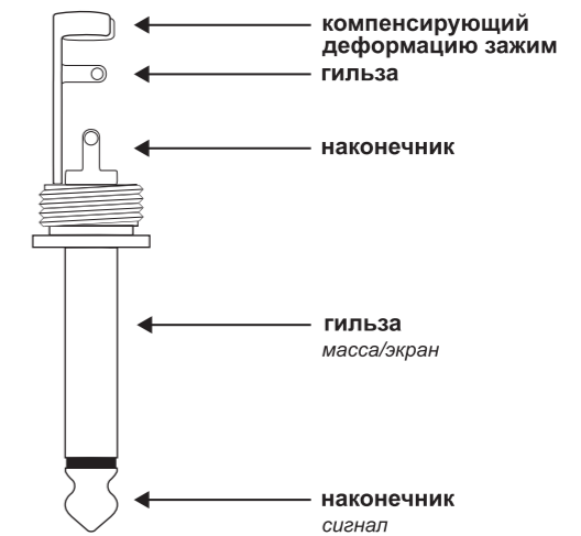
Рис. 3.2: 6,3-мм-монохраповый штекер
