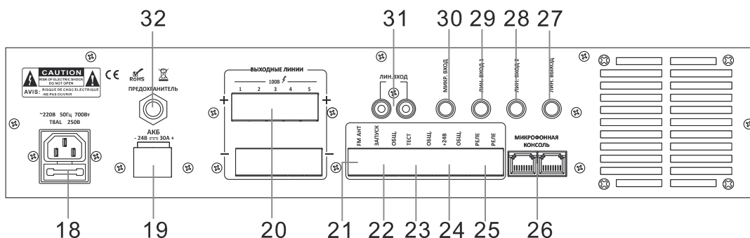
Рис. 1.3. Задняя панель
