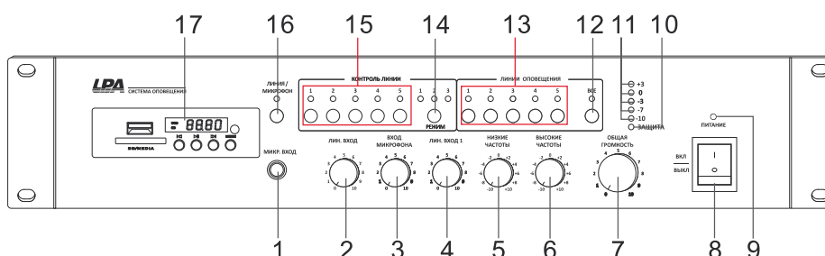
Рис. 1.2. Передняя панель
