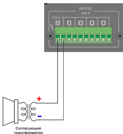
Рис. 2.2. Схема подключения громкоговорителей к LPA-TA-480MZ
